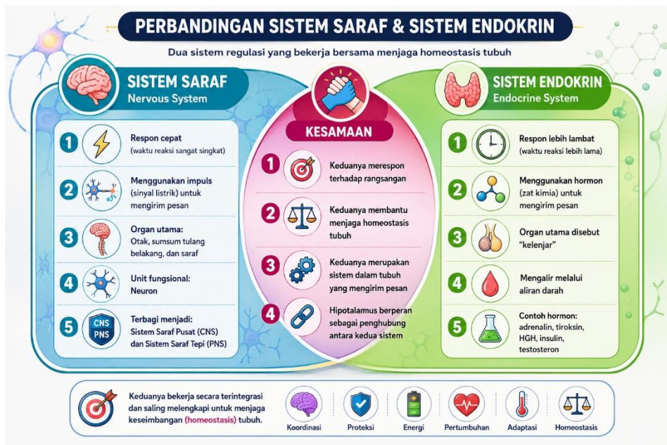
Gambar 4.1. Perbedaan antara sistem saraf dengan sistem endokrin
