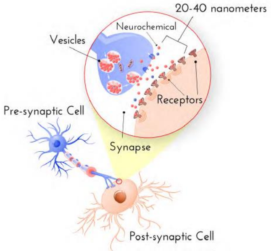
Gambar 3.2. Proses penghantaran sinyal saraf pada sinaps
